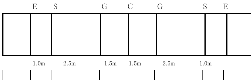
長さ10m(小学生3・4年生)のピスト図
